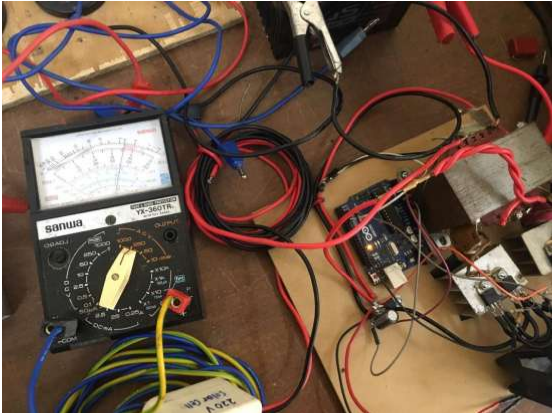
Lampiran 5. Proses pengujian dengan beban solder MASDA 40 Watt
