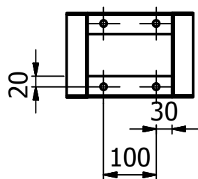
D-D ( 1 : 10 )
