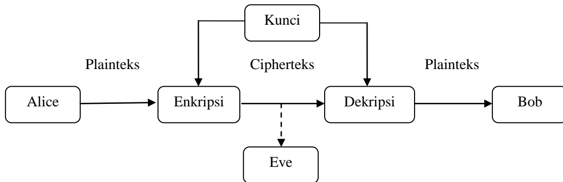
Gambar 1. Algoritma Kriptografi Simetris
