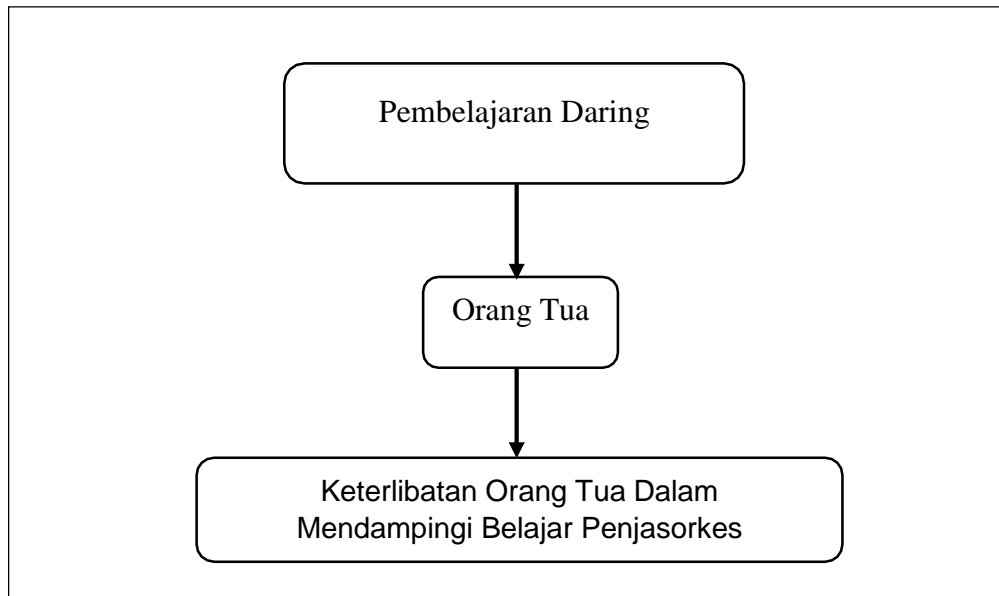
Gambar 1. 1 Kerangka Pikir
