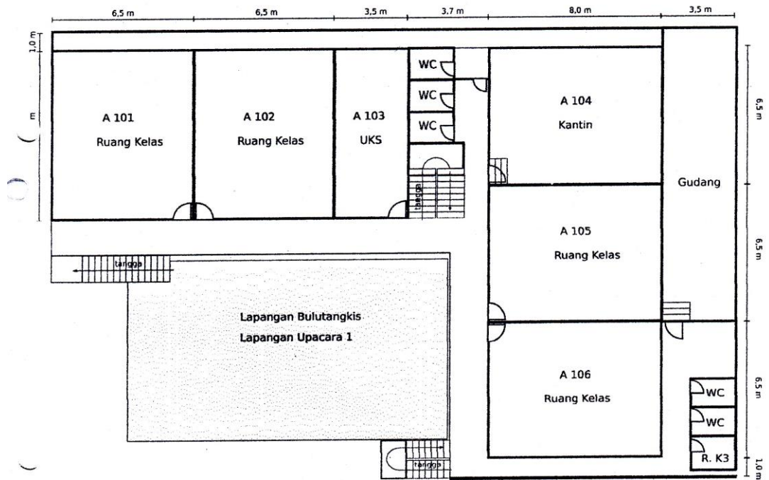
DENAH GEDUNG A LANTAI 1
