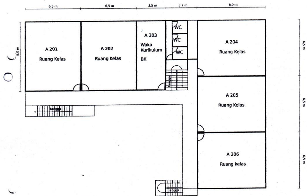
DENAH GEDUNG A LANTAI 2
