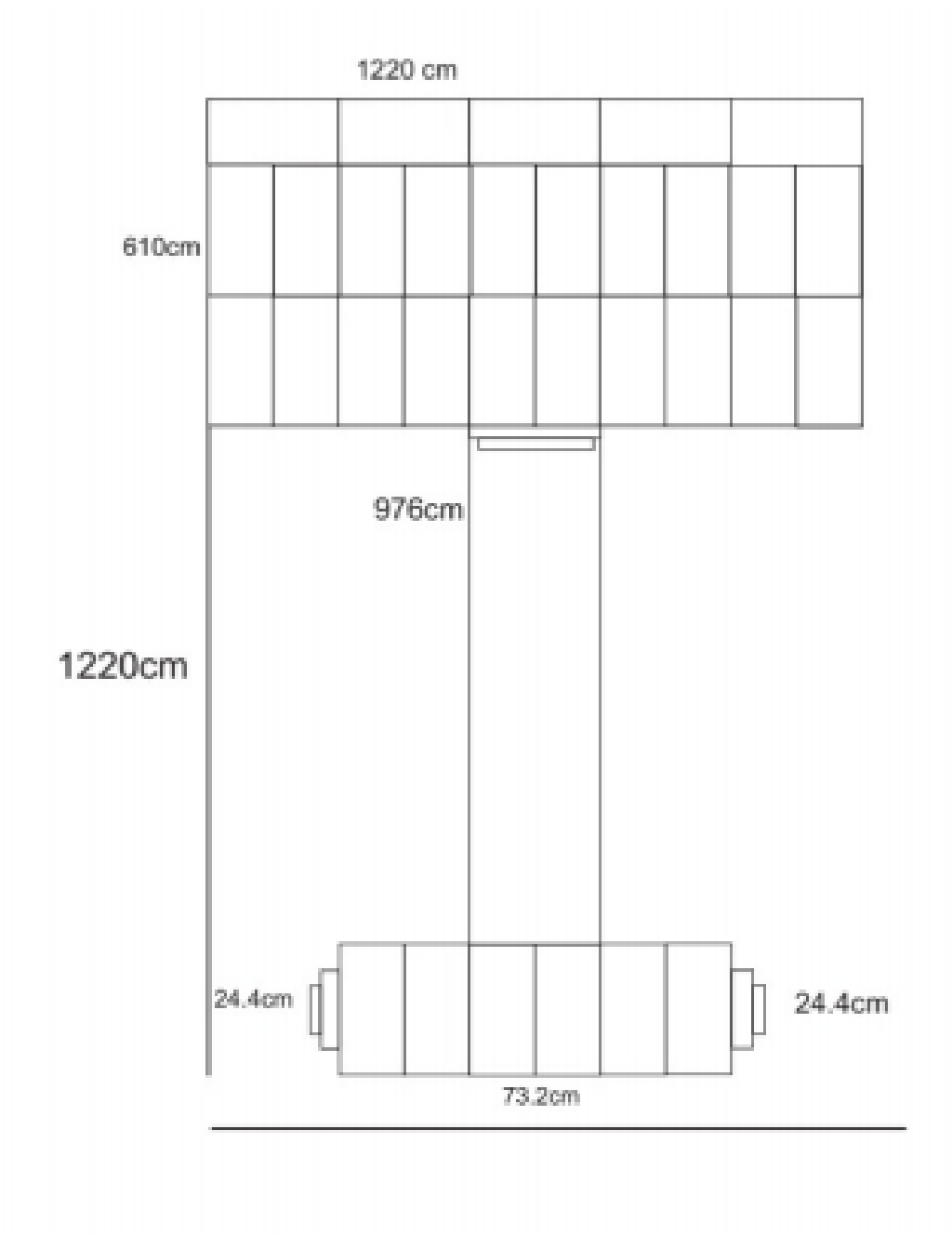
Lampiran 10. Ukuran Panggung
