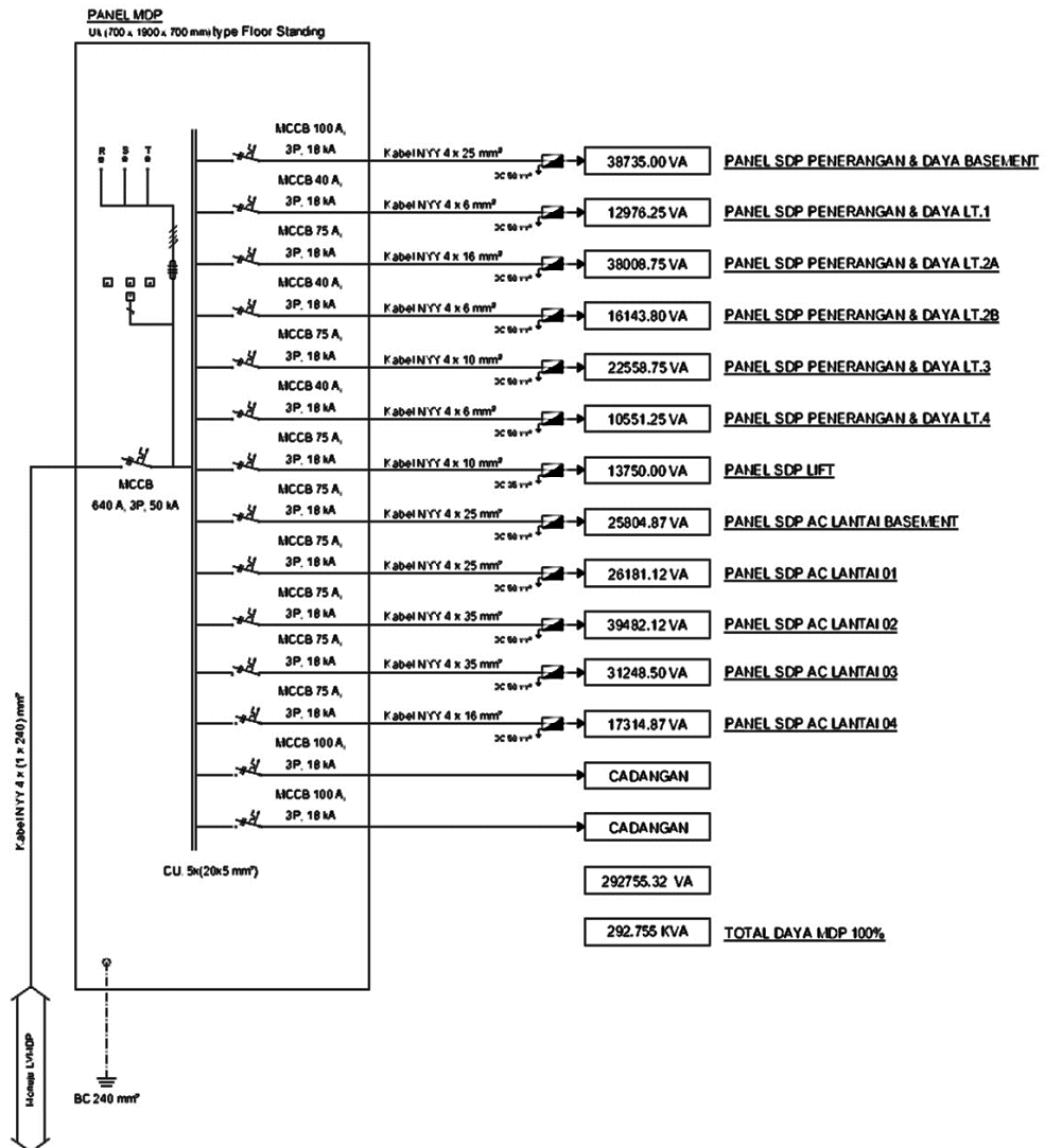
WIRING DIAGRAM MDP GEDUNG NTSC
