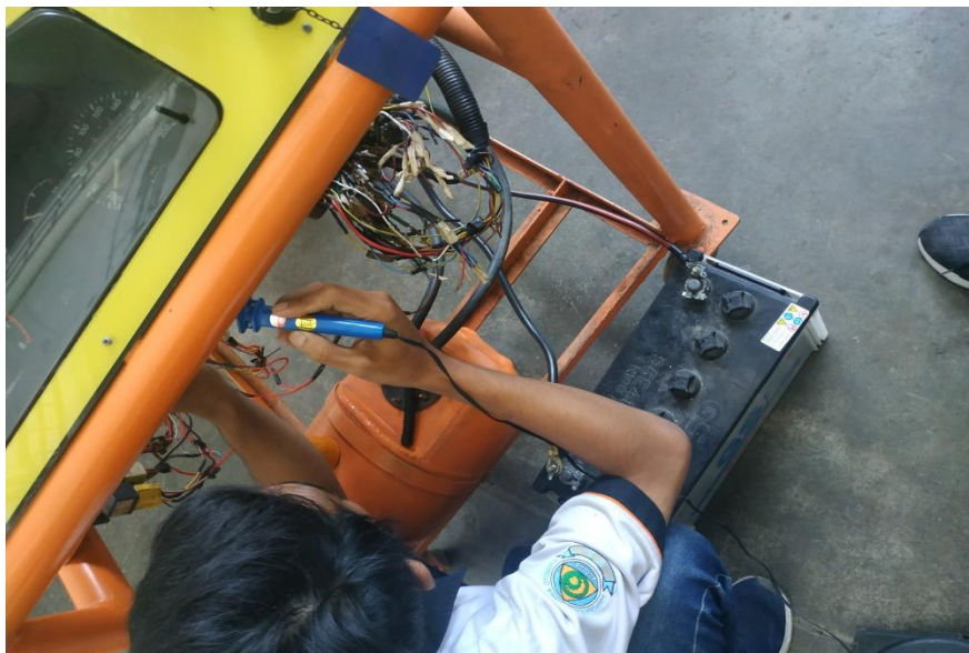
Proses pemasangan spedometer pada engine stand
