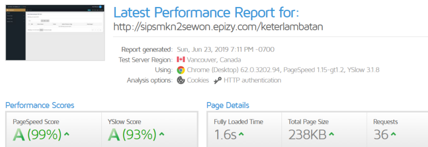
Gambar 74. Hasil Analisis GTMetrix pada Halaman Data Keterlambatan per Hari
