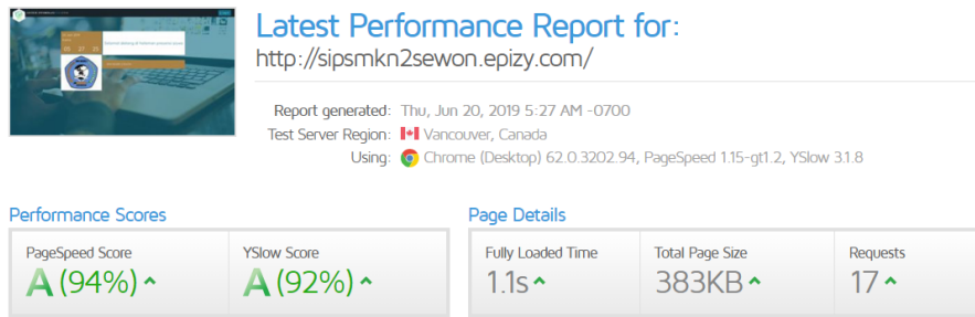
Gambar 64. Hasil Analisis GTMetrix pada Halaman Landing Page
