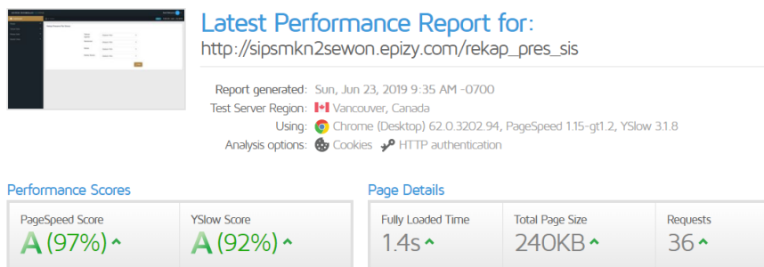
Gambar 77. Hasil Analisis GTMetrix pada Halaman Rekap Presensi per Siswa
