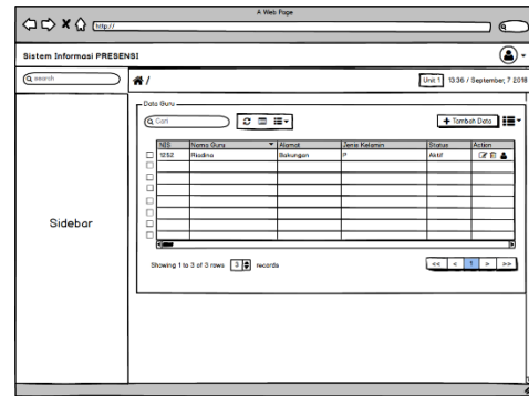
Gambar 37. Desain Halaman Data Guru
