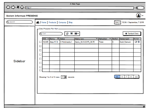
Gambar 22. Desain Halaman Perizinan per Hari
