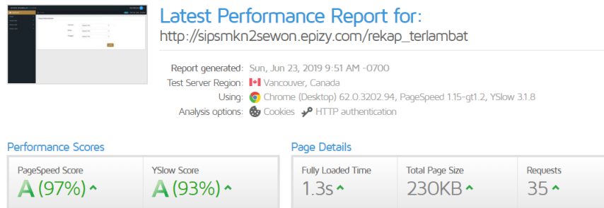
Gambar 80. Hasil Analisis GTMetrix pada Halaman Rekap Keterlambatan per Kelas
