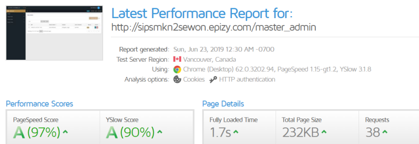
Gambar 86. Hasil Analisis GTMetrix pada Halaman Data Master Admin
