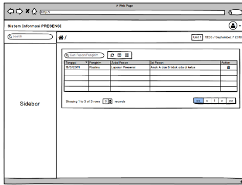
Gambar 19. Desain Halaman Pesan Masuk
