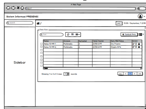
Gambar 41. Desain Halaman Data Kelas
