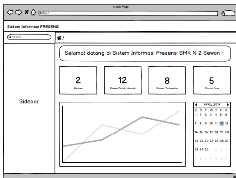
Gambar 15. Desain Halaman Dashboard
