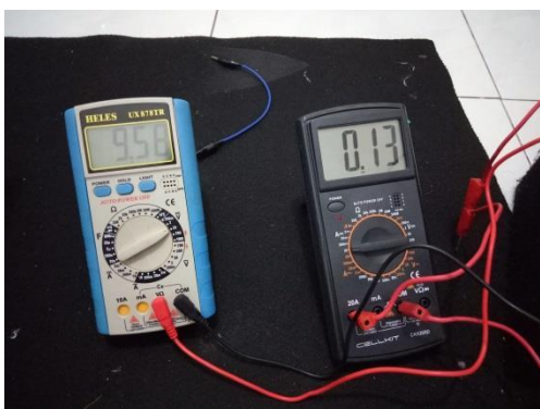
Lampiran 6. Pembacaan arus dan tegangan saat proses pengosongan ( discharging ) modul superkapasitor 80F/16.2V dan kelipatannya
