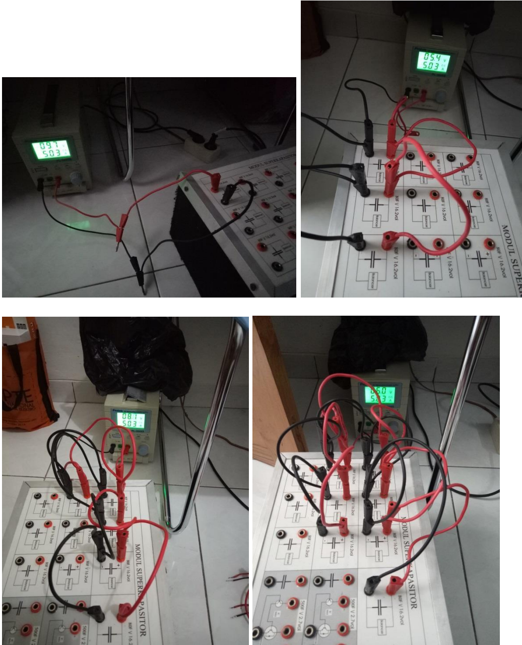
Lampiran 3. Proses pengisian ( charging ) modul superkapasitor 80F/16.2V dan kelipatannya
