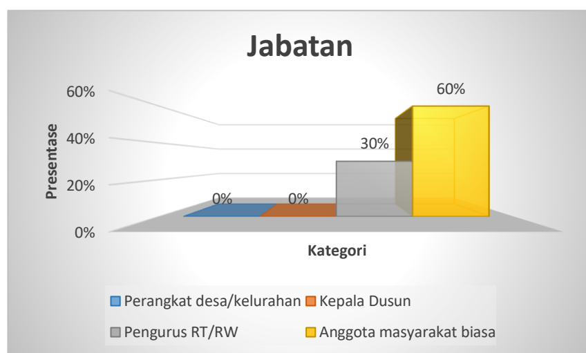
Gambar 29. Grafik Jabatan
