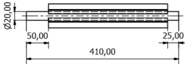
Gambar 2. Gambar kerja poros rol masuk kopi.
