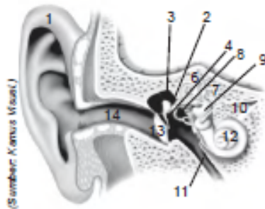
Gambar 1.20 Telinga beserta bagian-bagiannya. (1) Daun telinga, (2) Tulang martil, (3) Tulang landasan, (4) Tulang sanggurdil, (5) Tulang-tulang pendengaran, (6) Saluran setengah lingkaran bawah, (7) Saluran setengah lingkaran atas, (8) Saluran setengah lingkaran datar, (9) Saraf serambi, (10) Saraf rumah siput, (11) Tuba estachus, (12) Serambi, (13) Gendang telinga, dan (14) Liang dengar.
