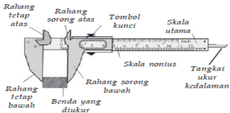
Gambar 1.2 Jangka sorong dan bagian-bagiannya.
