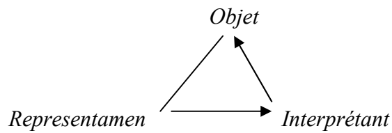
Gambar 2. Segitiga Triadik
