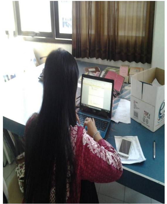
Gambar 3. Mengolah Data
