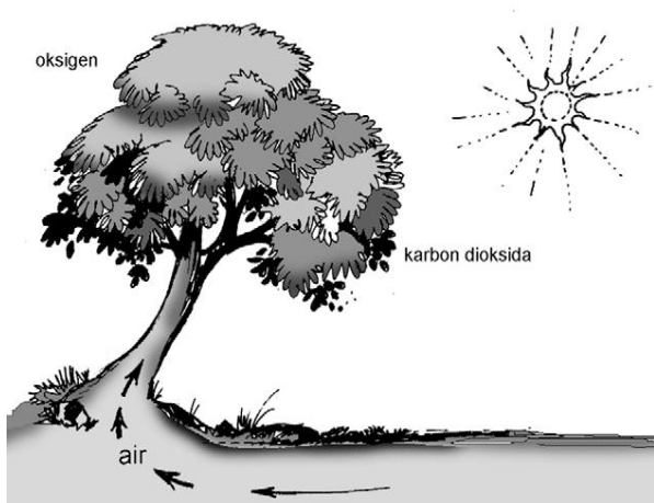
Gambar 1. Proses Fotosintesis
