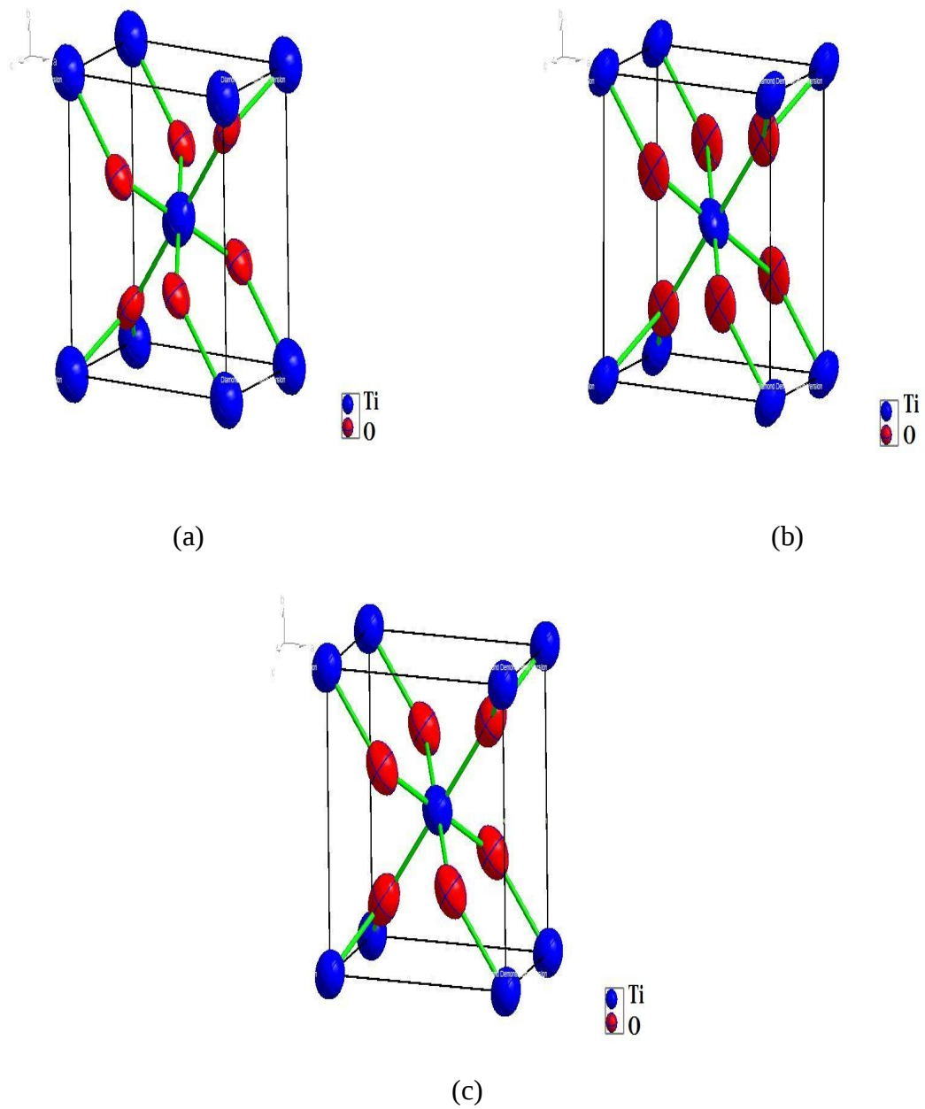
Gambar 7. Penggambaran struktur atom \text{TiO}_2 dengan faktor probabilitas (thermal ellipsoids) 80% pada variasi temperatur kalsinasi : (a) 500, (b) 700 dan (c) 900 °C
