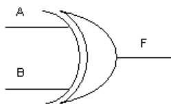
XOR
