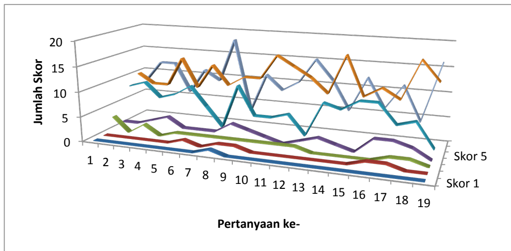
Gambar 30. Diagram Sebaran Skor Angket Usability
