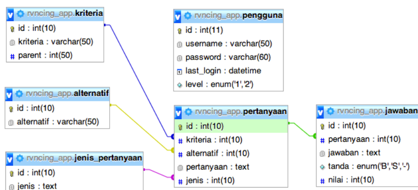
Gambar 18. ERD Database
