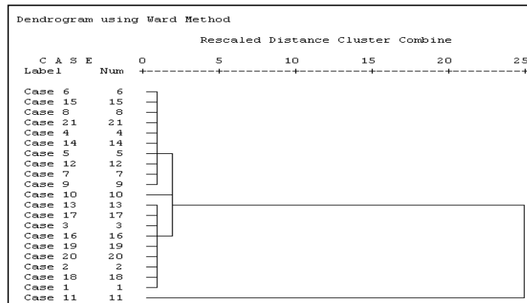
Gambar 2. Output Dendrogram Klaster Stasiun Curah Hujan Rata-Rata
