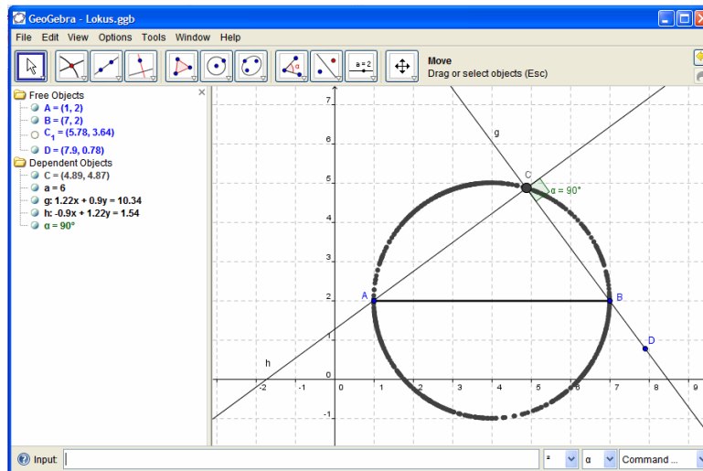
Gambar 4. Tempat Kedudukan
