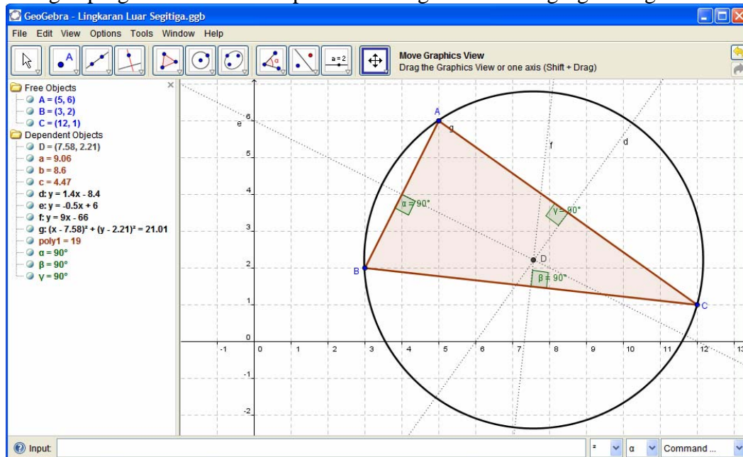
Gambar 2. Lingkaran-luar Segitiga
